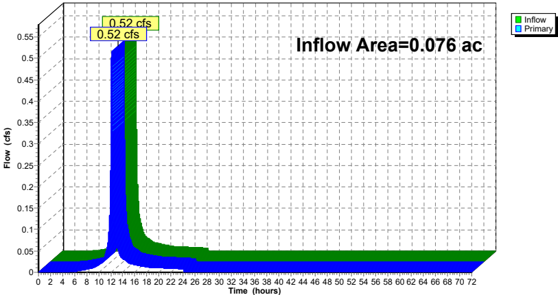
Link 6L: POI #3
