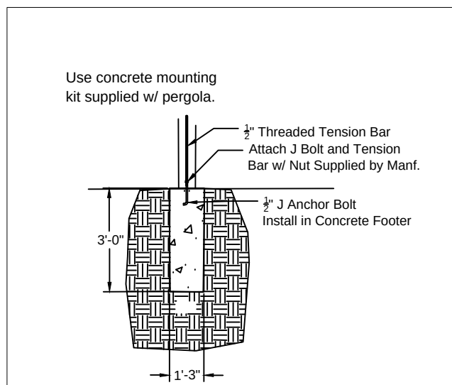
Pergola Footer Detail Scale: 1/4" = 1'=0"
